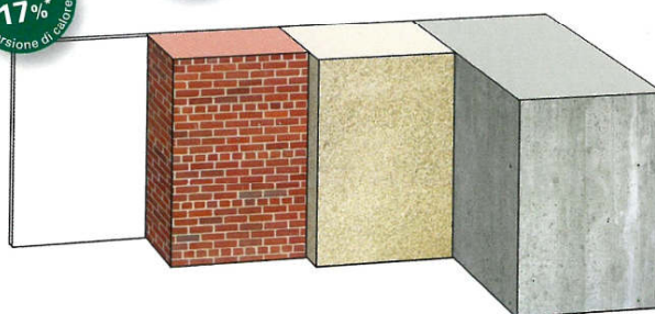
9 mm Depron pannello isolante 150 mm mattoni 203 mm arenaria 540 mm calcestruzzo normale
